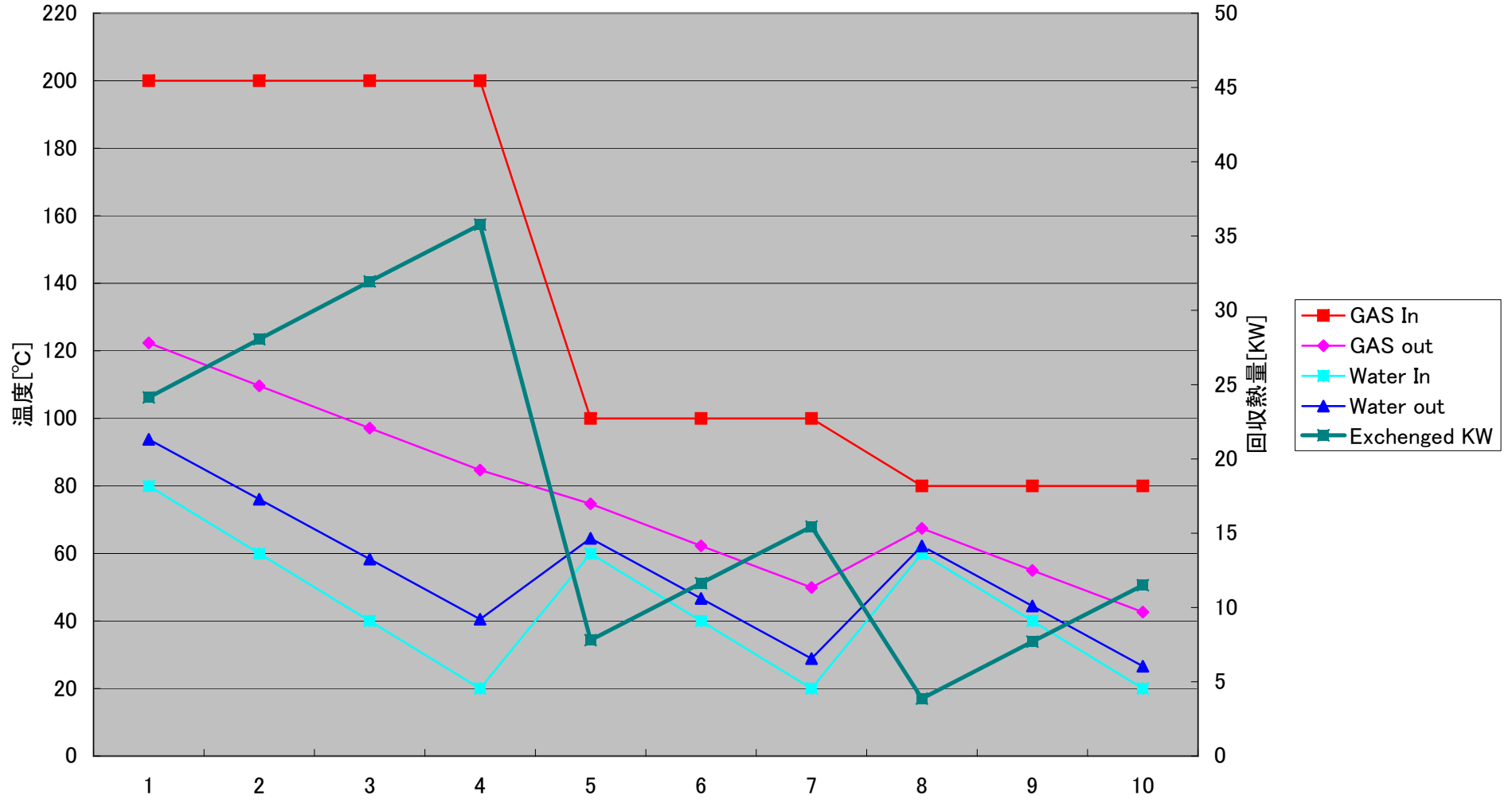
乾燥空気熱回収グラフ AIREC CROSS30-140 乾燥空気 1100kg/h(1163m 3 /h) & 水 1500kg/h
