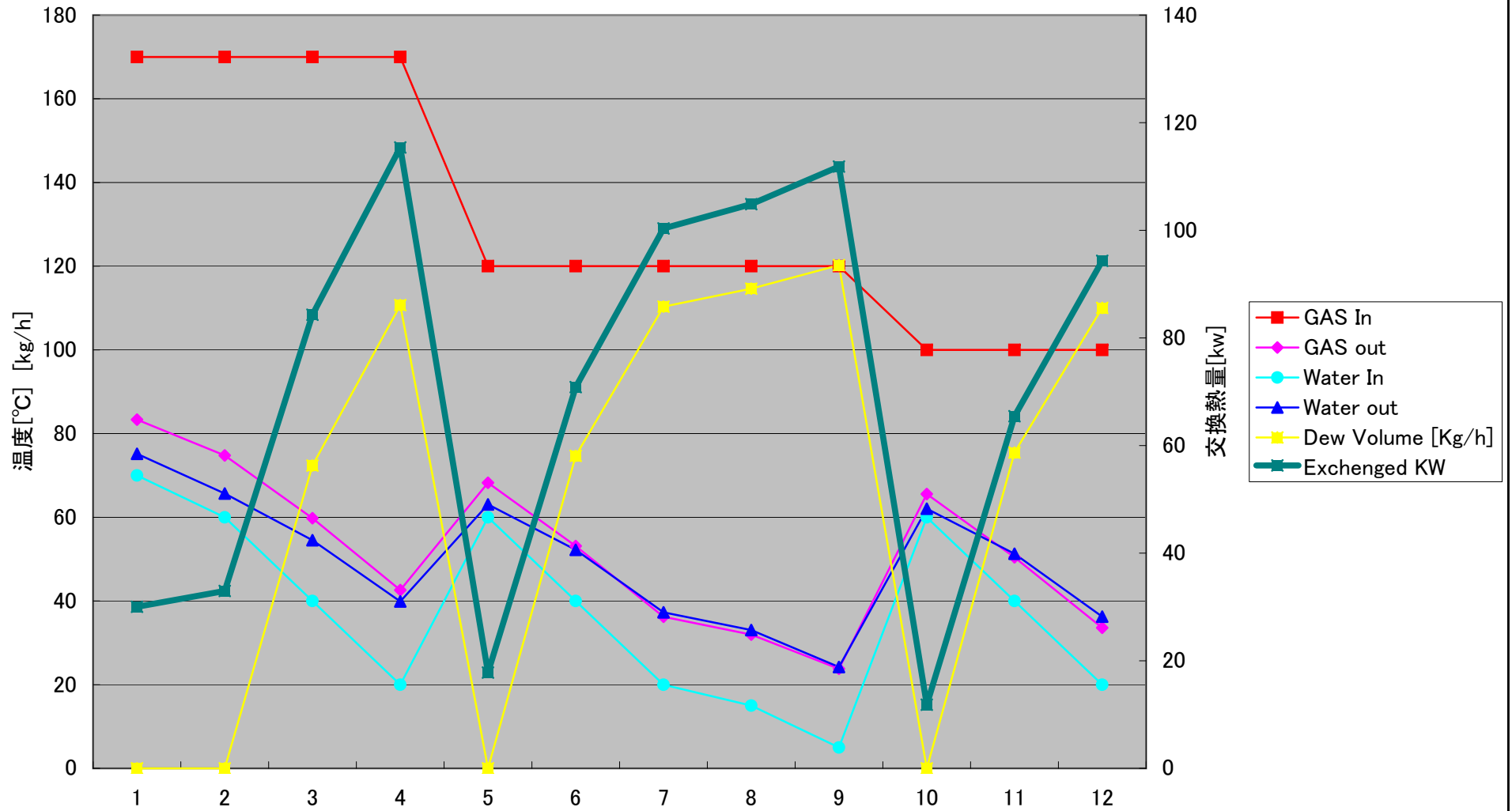
ガスボイラー排ガス熱回収グラフ AIREC CROSS30-140-2steps 排ガス 1100kg/h(1500m3/h) 絶対湿度0.1414kg/kg & 水 5000kg/h
